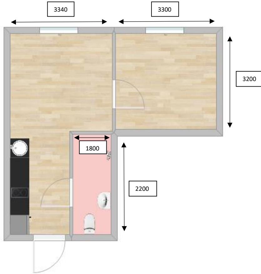
Rumsskiss 2-rums lägenhet
